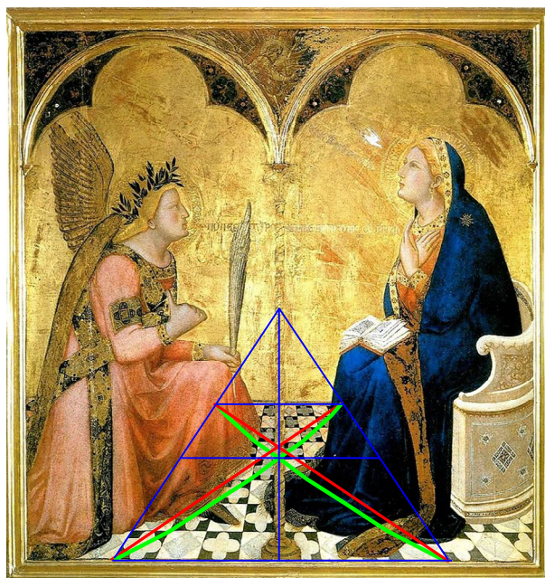
Рис. 23. Амброджо Лоренцетти. Благовещение . 1344. Красным цветом проведены прямые диагонали прямоугольника; зелёным — ломаные линии, составленные из диагоналей отдельных клеток.
