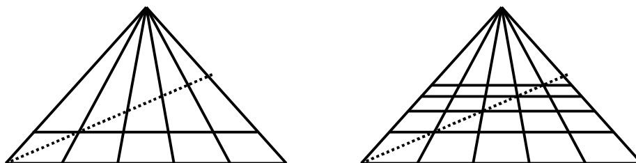
Рис. 24. Построение расчерченного на прямоугольники пола: (а) проведение первой и второй трансверселей, задающих направление вспомогательной диагонали; (б) проведение остальных трансверселей.
